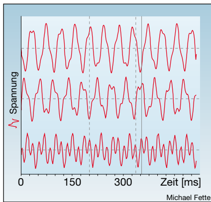
Bild 4 Signalmuster während des Blackouts in den USA 2003
