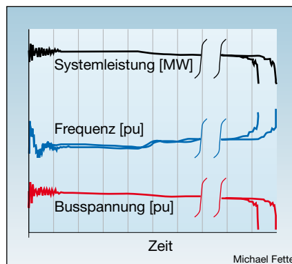
Bild 3 Langfristige Drift bis zum Kollaps
